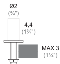
Cod. 332 Fissaggio tavolo Table mount Tischbefestigung
