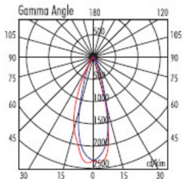
VAN 2 - MR16 - 50W 38°
