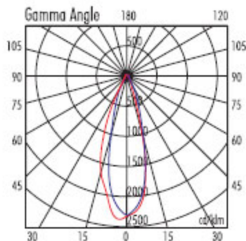
IGEA 2 - MR16 - 50W 38°
