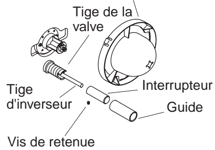
Ensemble inverseur
